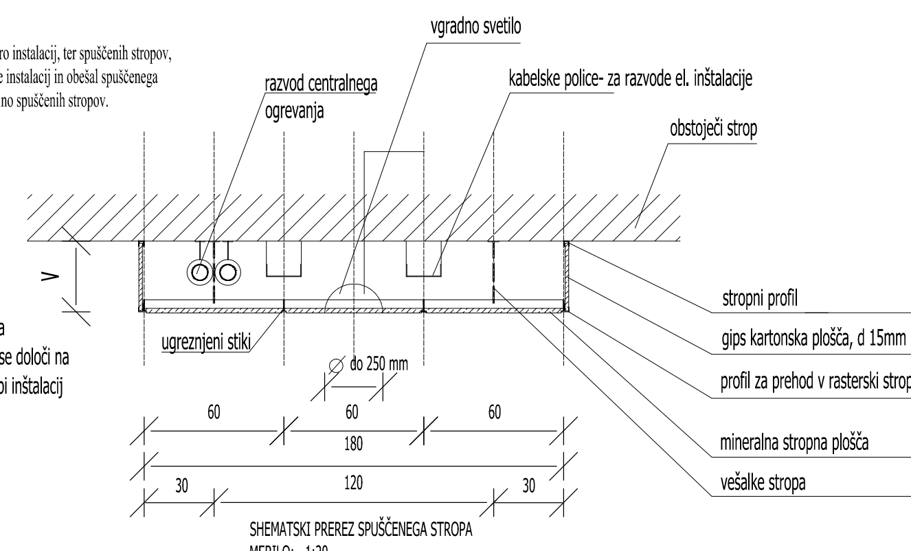
SHEMATSKI PREZEV SPUŠČENEGA STROPA MERILO: 1:20
