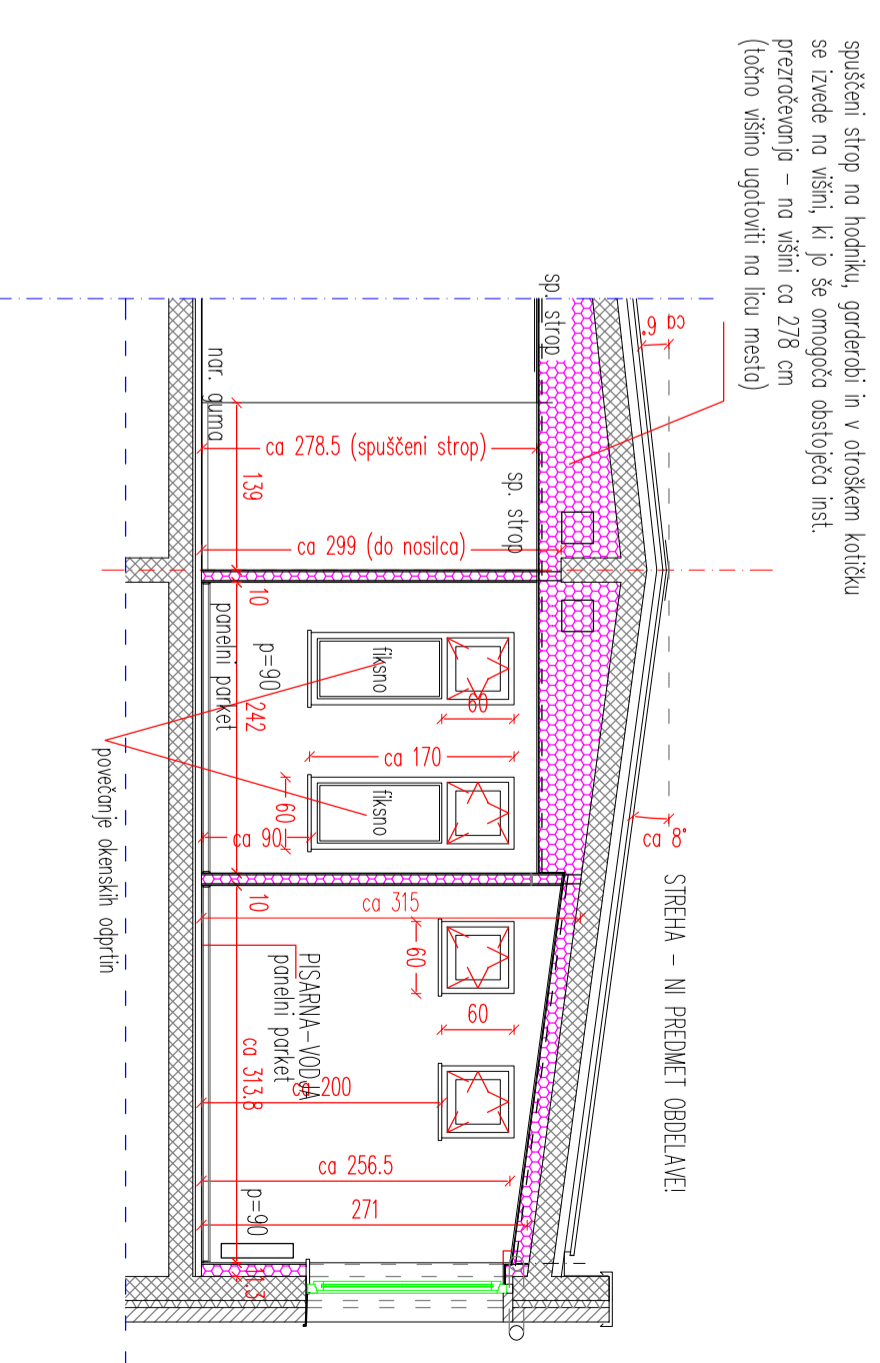
DELNI PREREZ B-B; 1. nadstropje
